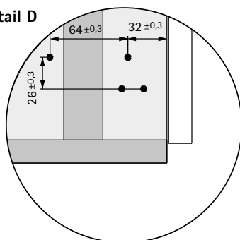
Schnitt C-C
