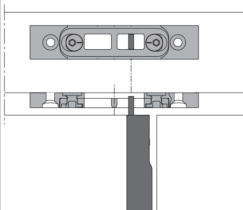
2 flg. Fenster mit 1 Riegel
