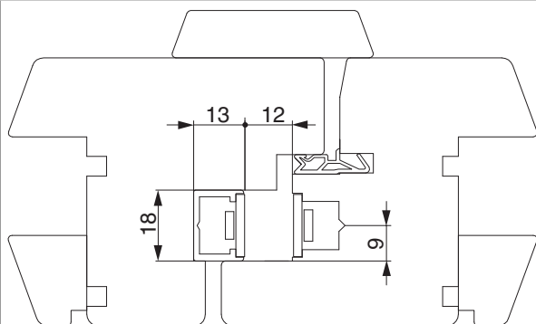
Stulp 18mm Falztiefe glatt
