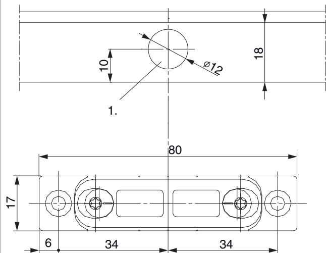
Riegelschließteile mit Positionzapfen
