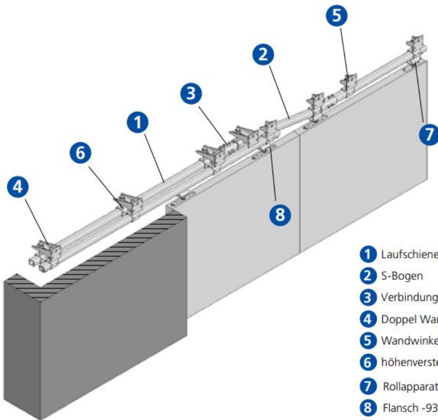
Abbildung 2. Einbaubeispiel
