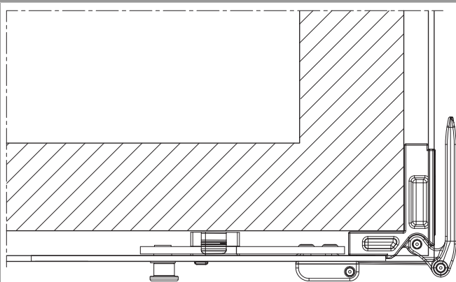
Flügel in Geschlossen-Stellung
