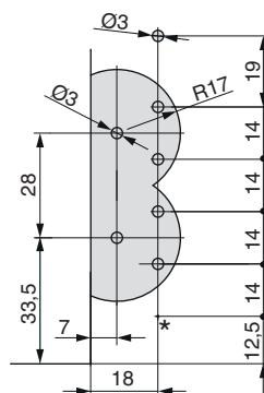
12/18 für Fenstertüren
